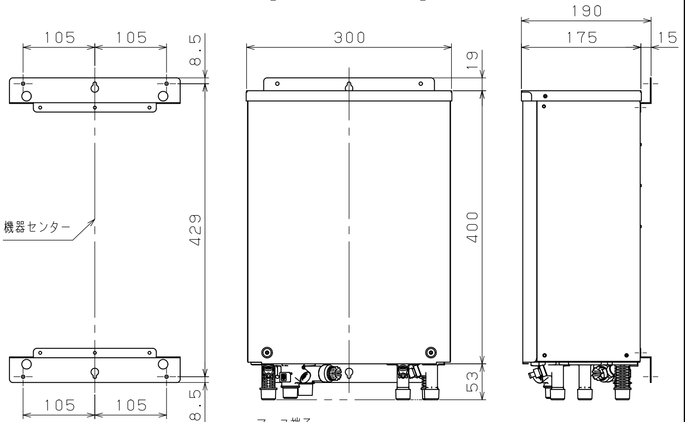
【取付寸法（機器前面より）】
